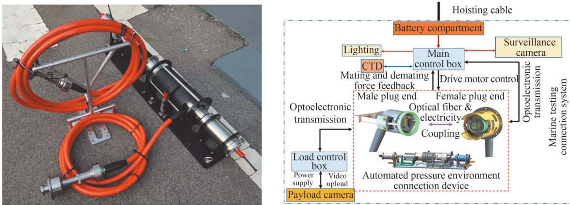
图2 自动接驳装置及海试接驳系统原理图
