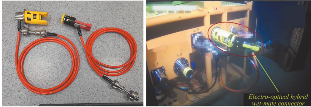
图1 水下插拔光电连接器样机及1 625米深海试
